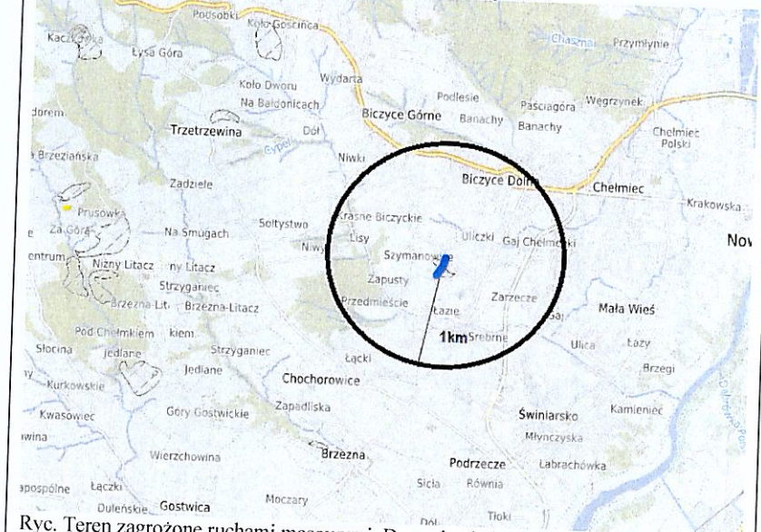
Ryc. Teren zagrożony ruchami masowymi. Dane sip.chelmiec.pl
